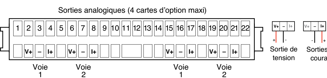
Figure 2.2.1d Câblage des options page 1
