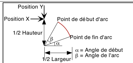
Figure 7.4.20a Définition des dimensions d'un arc
