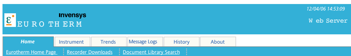
Figure C1 Page d'accueil
